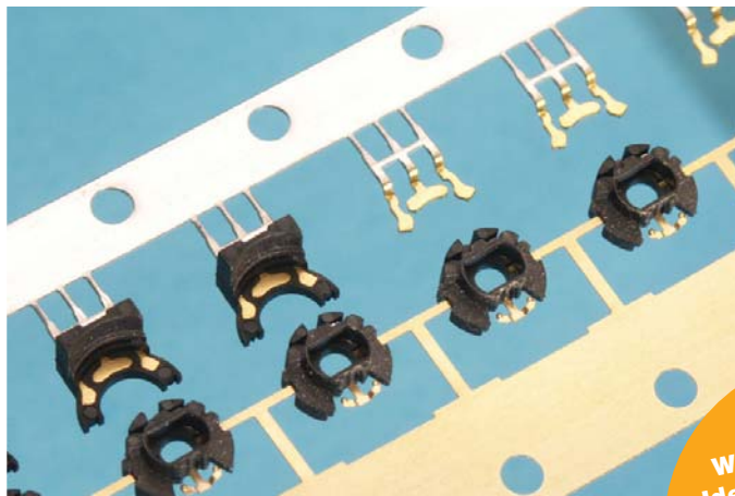
Hochpräzise umspritzte Kleinteile auf partiell vergoldetem und verzinnem Stanzband
