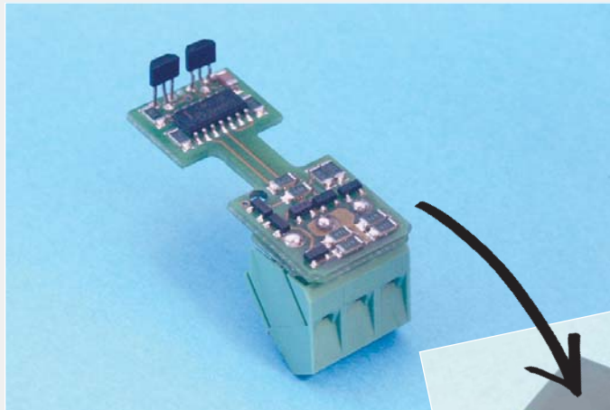
Leiter-Platte mit zwei Hallsensoren und Auswertungselektronik wird umspritzt und ist nun bereit für den harten Dauereinsatz
