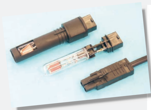
Kundenspezifische Sonderstecker mit integrierten Sensoren, komplett bei Satrotec hergestellt.
