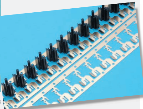
Beispiele umspritzter Stanzbänder, die bei Satrotec gefertigt werden.
